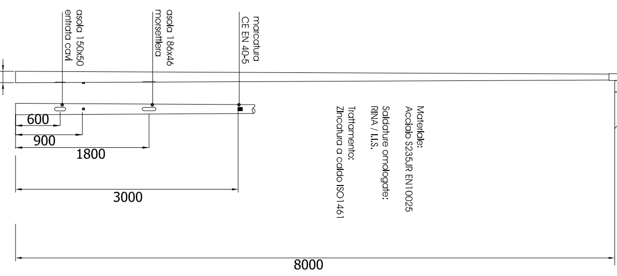
Particolare apparecchi ill. esterni
